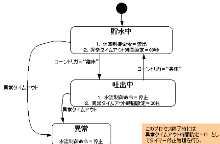
PSEPC1.2 水はね防止運転の状態モデルによるプロセス仕様
