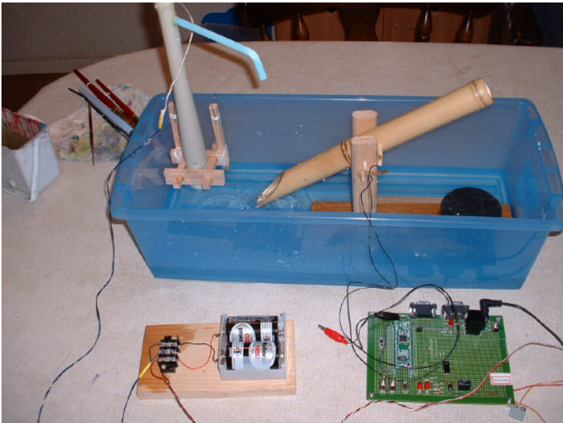
動作中の鹿脅し
